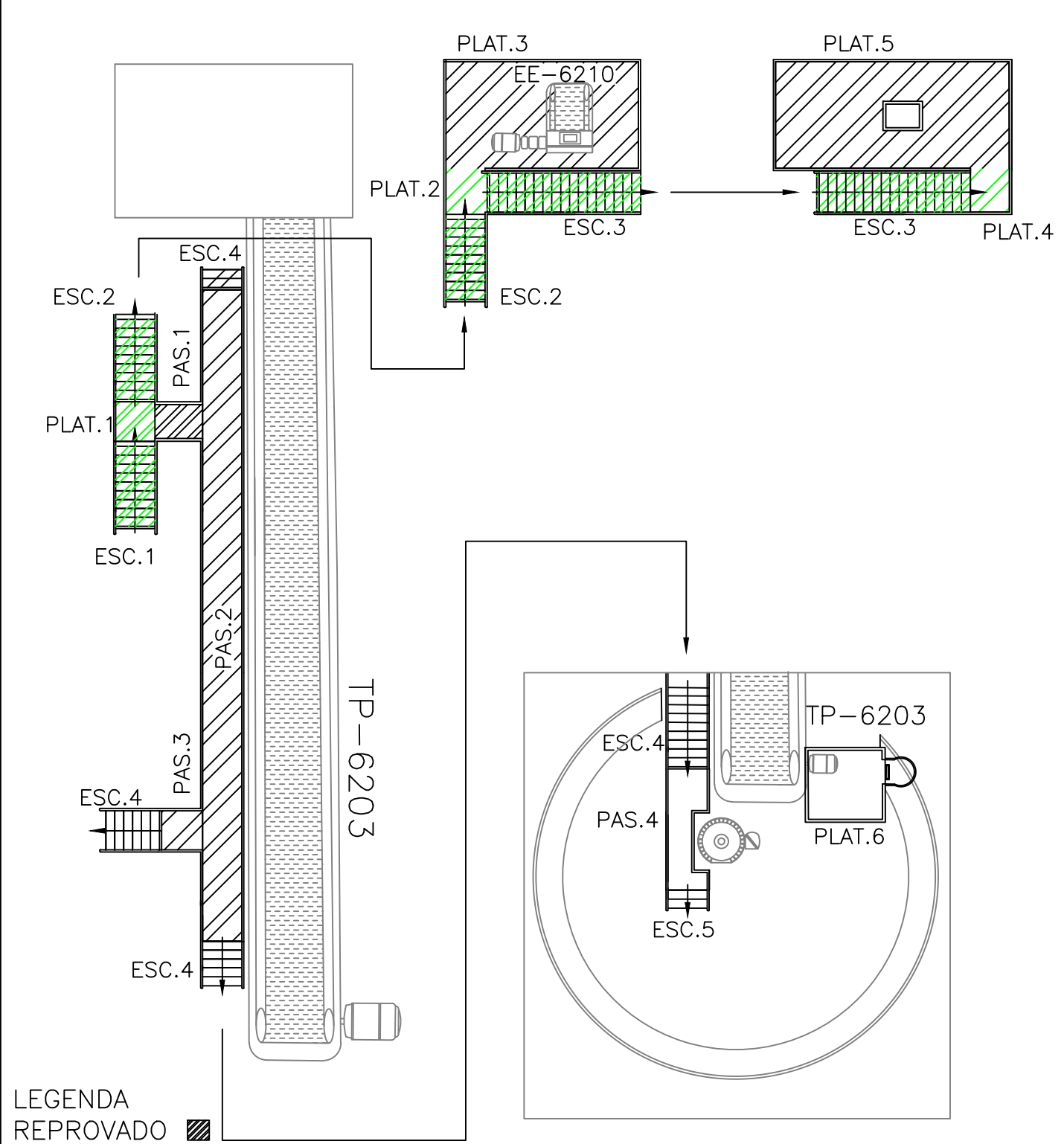
DESENHO 47 - U-620 - TP-6203 / EE6210
