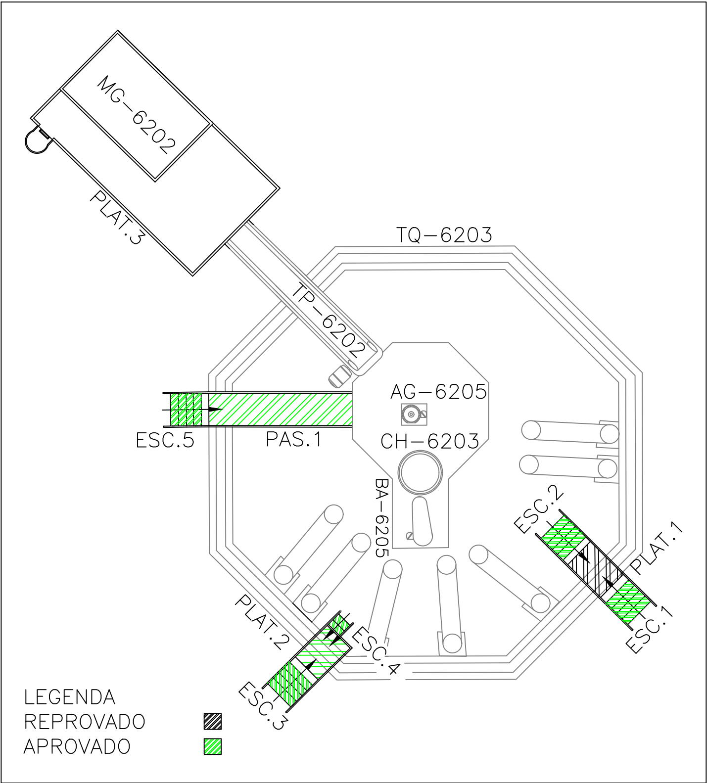
DESENHO 48 – U-620 – BA-6205 / AG-6205
