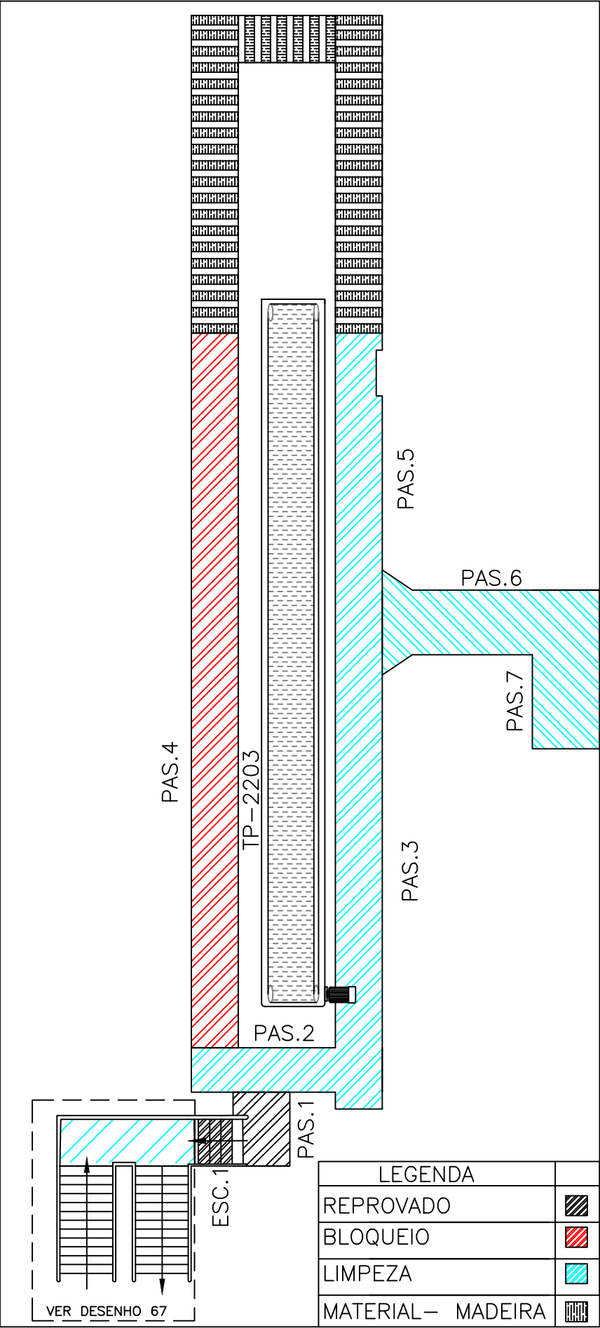
DESENHO 64 – 3º PATAMAR U220 TP2203
