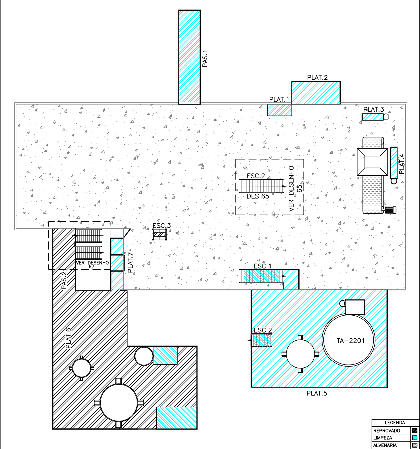
DESENHO 66 – U220 – TP-2201(TERREO) – TA-2201
