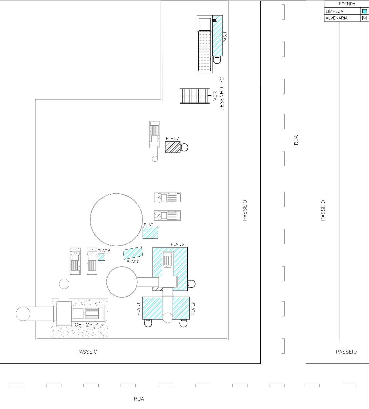
DESENHO 73 – U-260 CB-2604
