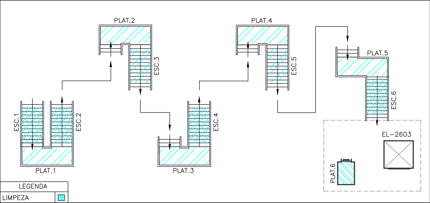
DESENHO 82 – U260 – ACESSO AO EL-2603
