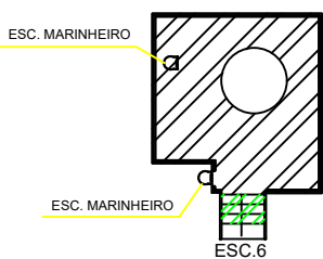
5° PLATAFORMA/PATAMAR
