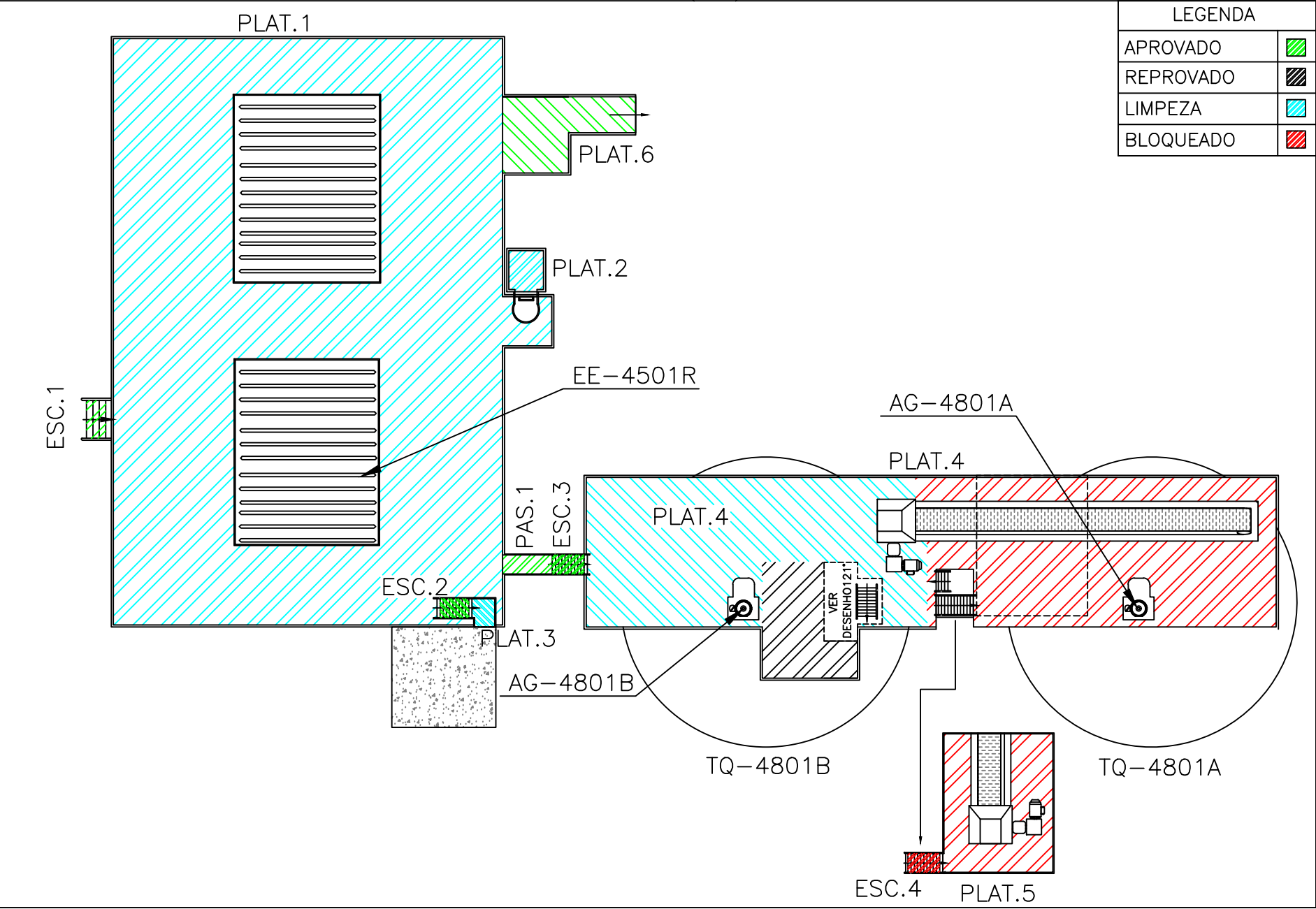
DESENHO 120 – EE-4501R – PLAT.SUPEIOR TQ-4801(A,B)
