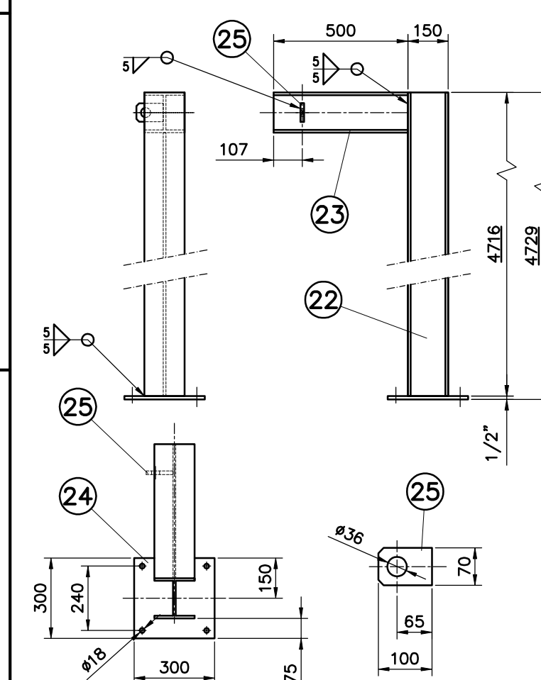
ANCORAGEM 03 CONJUNTOS
