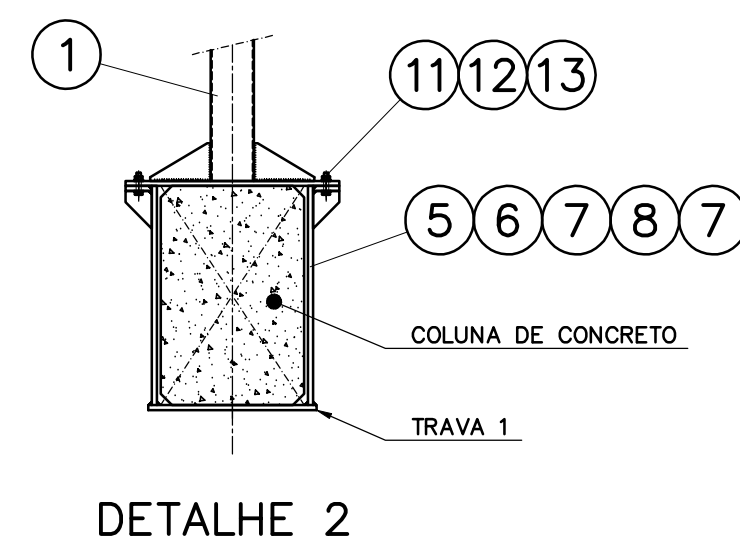
DETALHE 2
