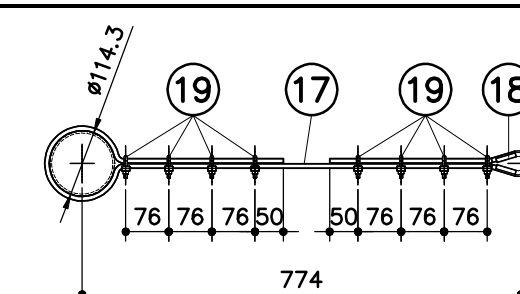
ANCORAGEM 03 CONJUNTOS
