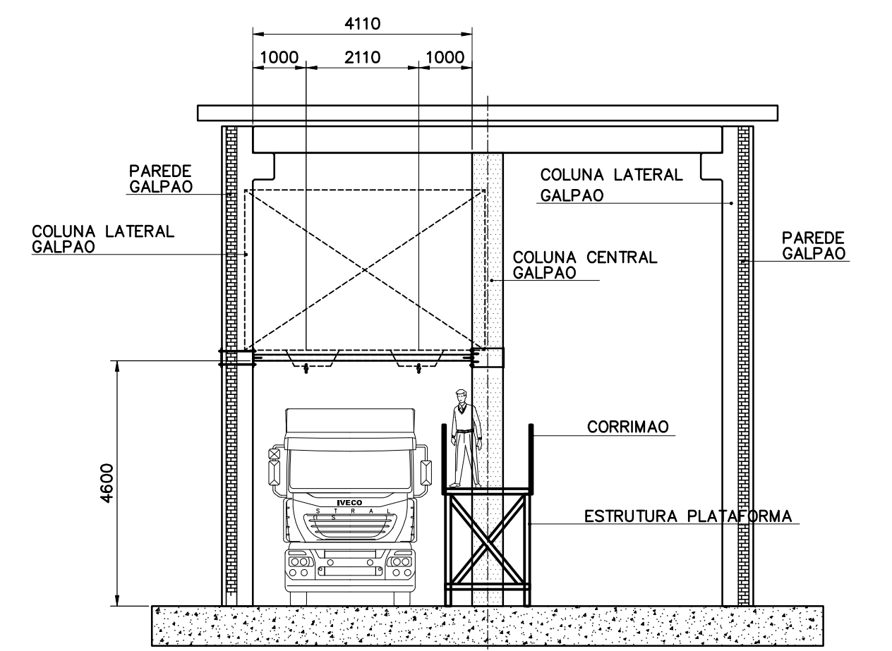
CORTE BB
