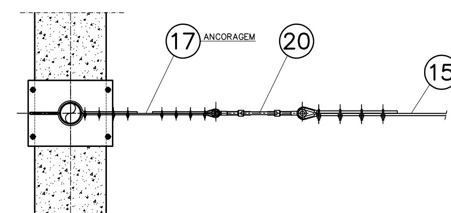
DETALHE 3
