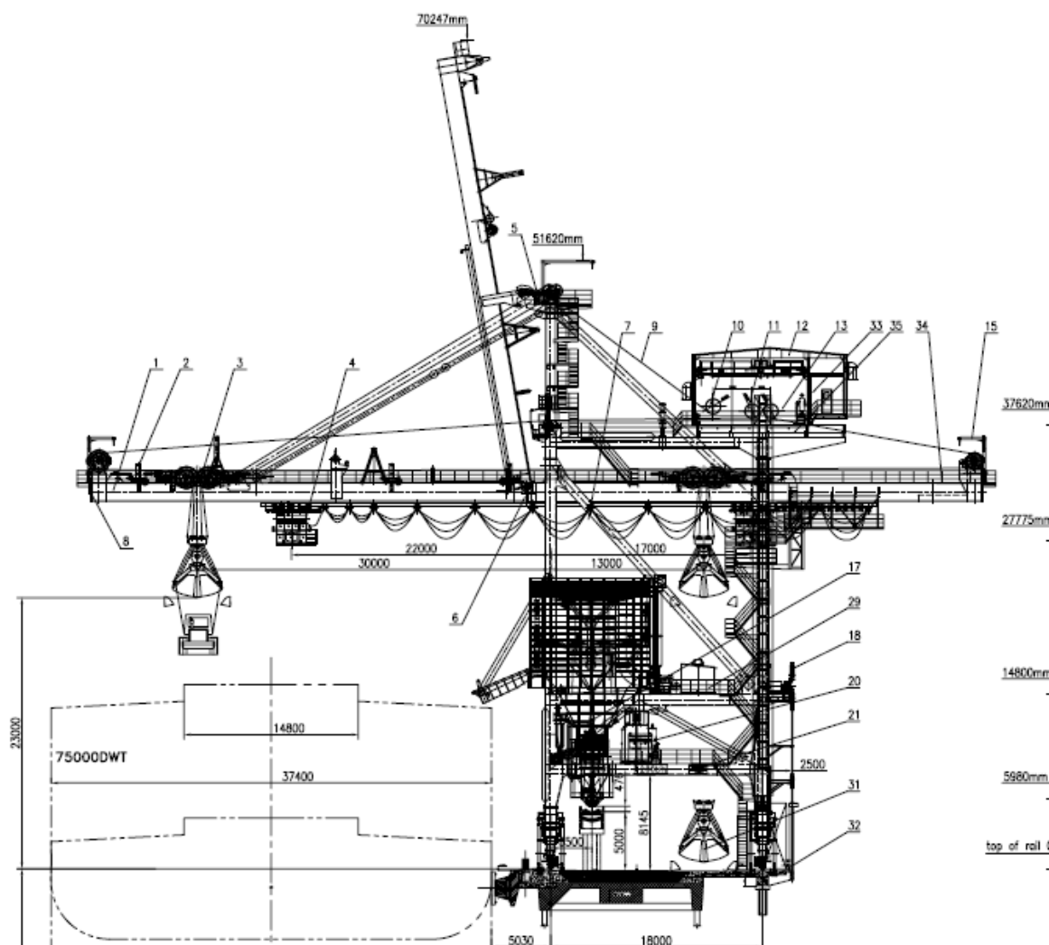
DESENHO DO DESCARREGADOR DE NAVIO
